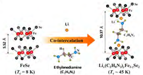
Fig. FeSeへのLiとEthylenediamineのコインターカレーション(共挿入)。
