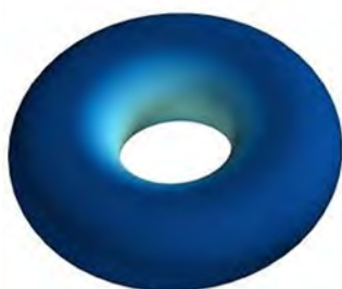
:楕円曲線 y^2 = x^3 + ax + b
